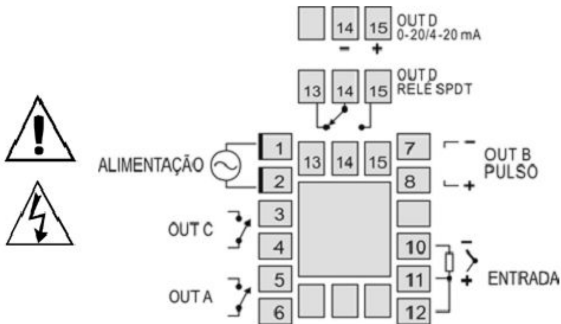
Fig. 1 - Ligações elétricas do controlador
